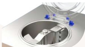
Cuve ouverte et bras de mélange
